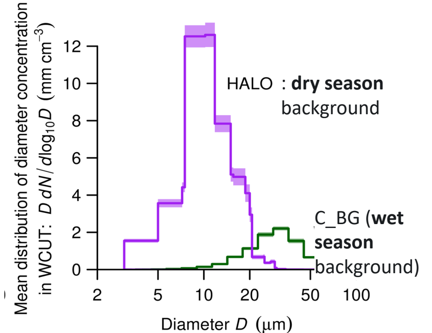
Droplet SD (Romps23)
